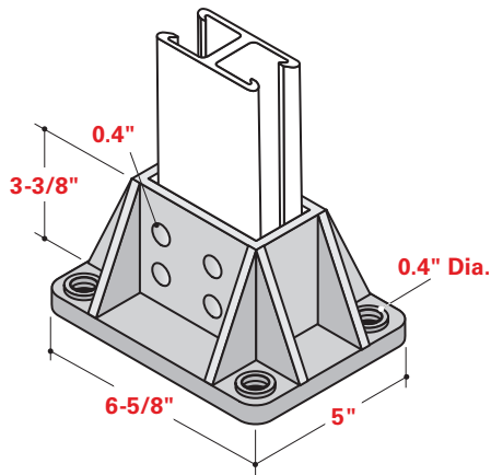
CS-PB-20D (1-5/8" x 3-1/4"), CS-PB-10D (1-1/8" x 2-1/4")
