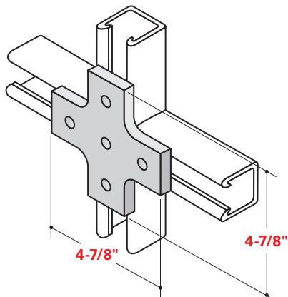
CS-2518P, CS-2518V
