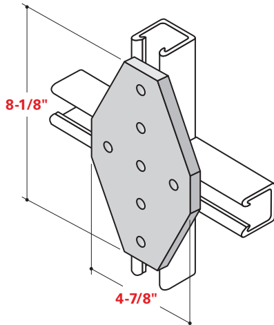
CS-2534P, CS-2534V
