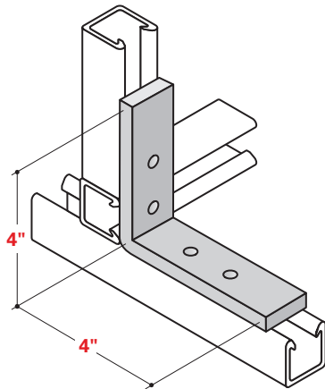
CS-2541P, CS-2541V
